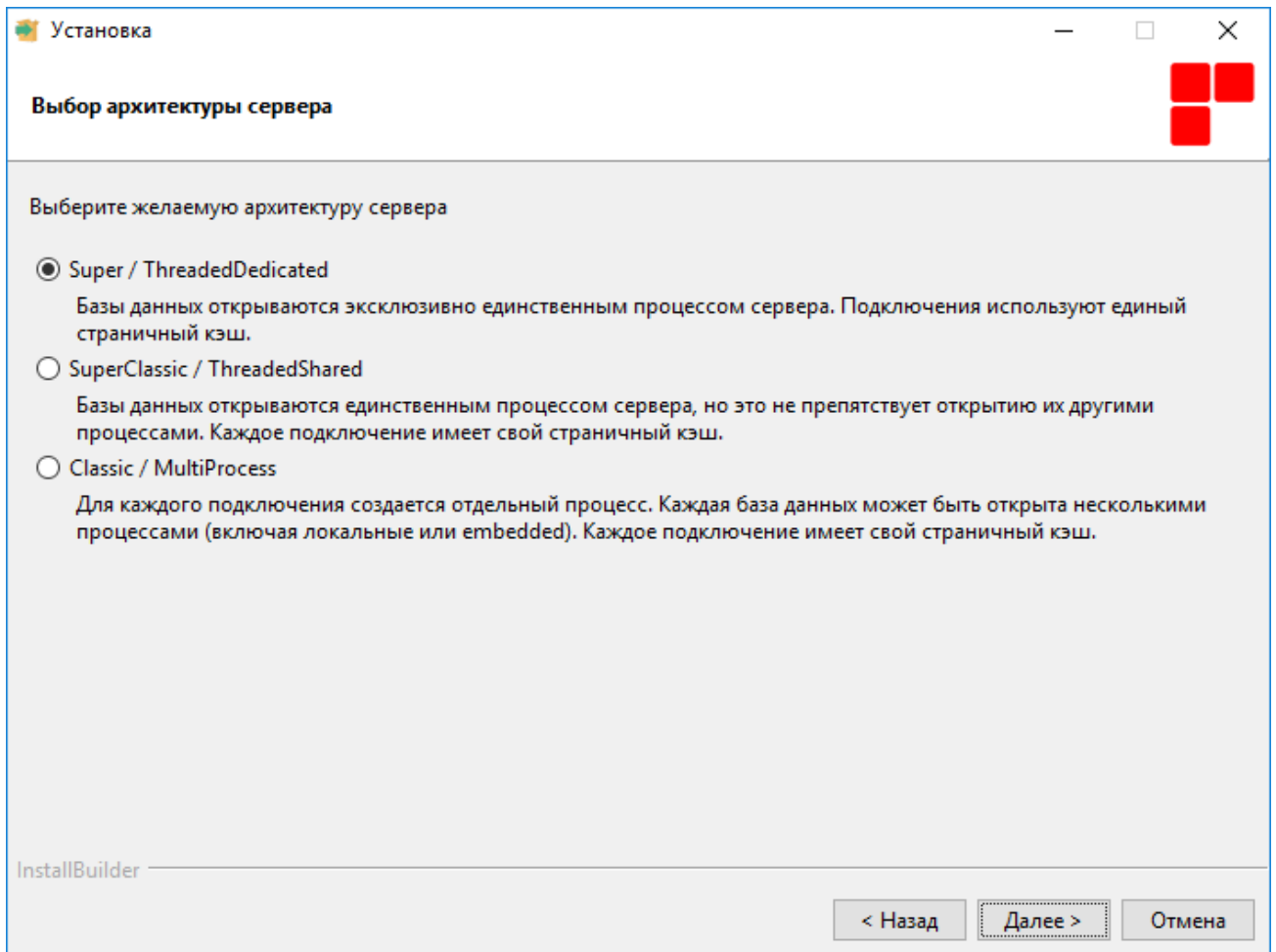
Рис. 12 – Выбор архитектуры сервера СУБД «Ред База Данных»
